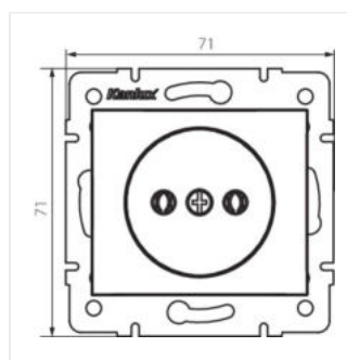
DOMO 01-1210-142 cm
