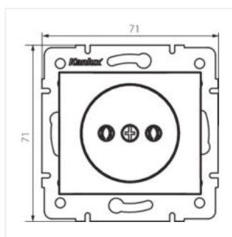
DOMO 01-1210-130 pe
