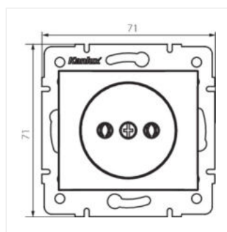
DOMO 01-1210-150 sz
