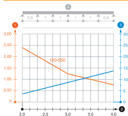
Zatěžovací diagram kabelového žlabu typu SKSMU 110
