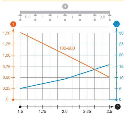
Zatěžovací diagram kabelového žlabu typu MKSU 60
