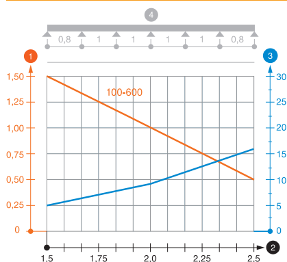
Zatěžovací diagram kabelového žlabu MKS 60 VA
