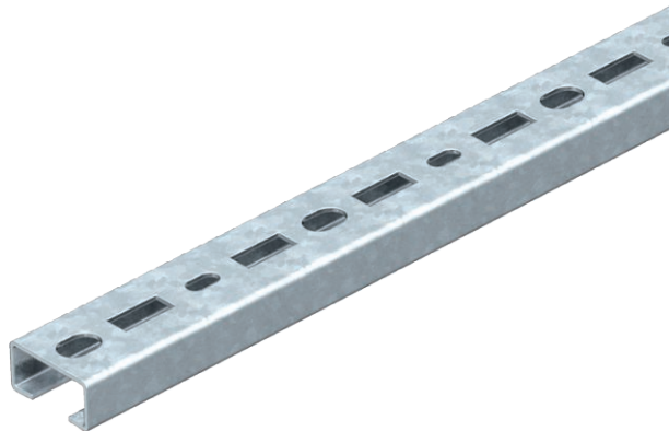
Profilová lišta děrovaná, šířka výřezu 16 mm.
