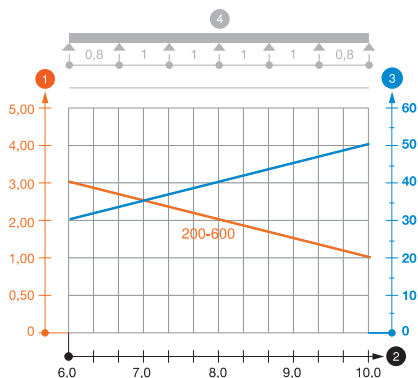
Zatěžovací diagram kabelového žebříku pro velká rozpětí typu WKL 200
