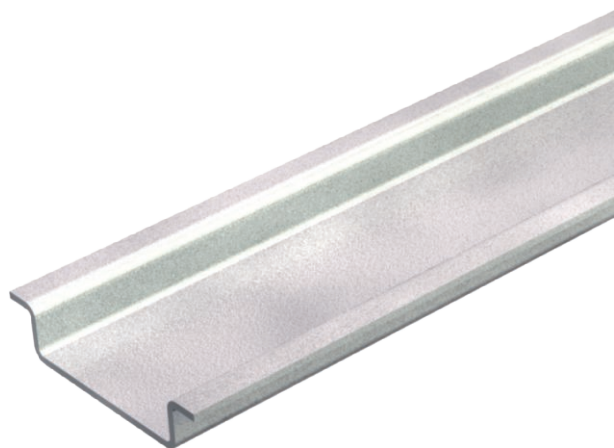
Přístrojová lišta 35 × 7,5 mm dle EN 60715 (dříve EN 50022).
