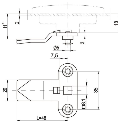
Jazýček 3 bodový se zarážkou, s pojistnými kroužky
