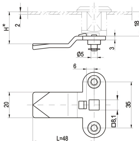
Jazýček 3 bodový se zarážkou, s pojistnými kroužky
