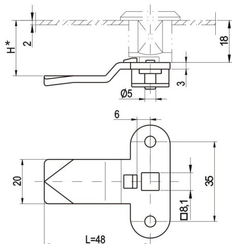
Jazýček 3 bodový se zarážkou, s pojistkou
