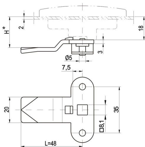
Jazýček 3 bodový se zarážkou, s pojistkou
