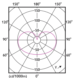
LEDcandle MAS B35 3,4W E14 927 FR-LDD
