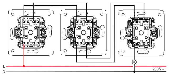
Permutateur
