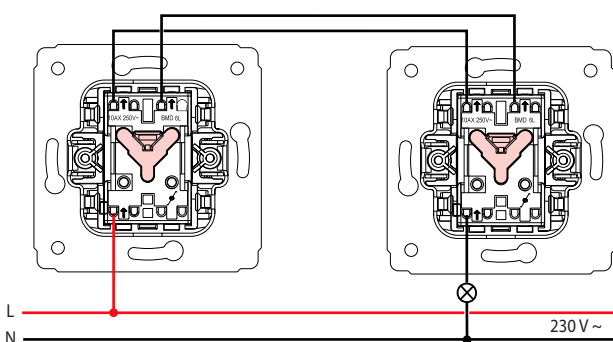
Va-et-vient lumineux
