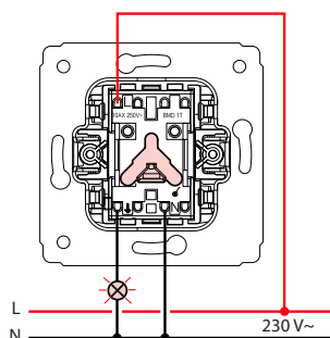
Interrupteur simple témoin
