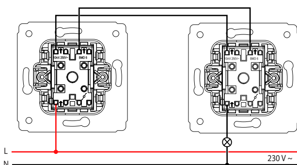
Va-et-vient
