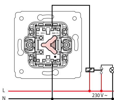
Poussoir lumineux
