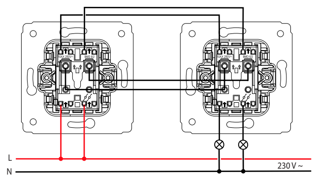
Permutateur
