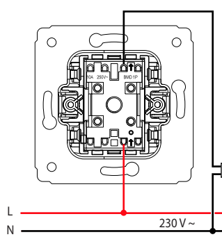
Poussoir
