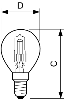
HalClass 18W E14 230V P45 CL
