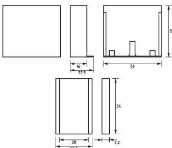
Maßzeichnung Gruppenansicht
