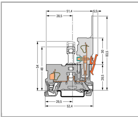
Trennbasisklemme
