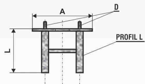
ZÁKLADOVÝ RÁM ZR 300 KKA P
