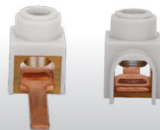
Připojení do přístrojů pomocí konektoru kolík (jazýček)
