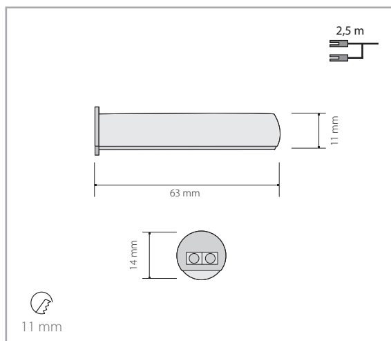
Senzor SL6001 - POHYBOVÝ | MOTION BEWEGUNGSSENSORAUSSCHALTER
