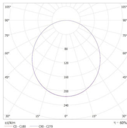
KANLUX S.A. (kat 38779) BENO 24-30W CCT-L G 30W / Krzywa rozsyłu światła (biegunowo)
