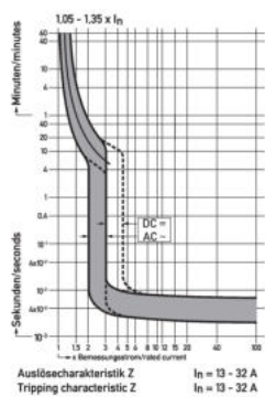
Diagramme Leitungsschutzschalter DLS 6i, Z-Charakteristik, 10 kA
