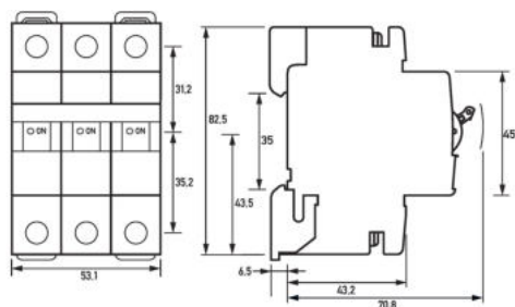
Maßzeichnung Leitungsschutzschalter DLS 6i, Z-Charakteristik, 10 kA
