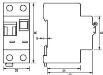
Maßzeichnung FI-/LS-Kombinationen DRCBO 3 Typ AC, B-Charakteristik, 1+N-polig
