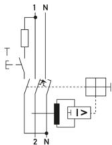
Schaltungsbeispiel FI-/LS-Kombinationen DRCBO 3 Typ AC, B-Charakteristik, 1+N-polig
