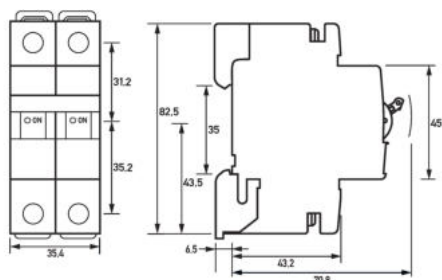
Maßzeichnung Leitungsschutzschalter DLS 6i, Z-Charakteristik, 10 kA
