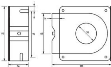
Maßzeichnung Gruppenansicht
