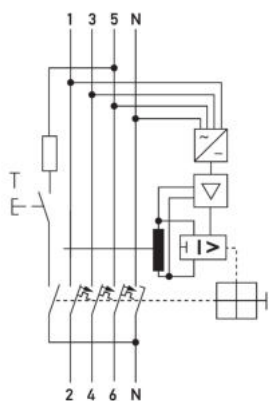
Schaltungsbeispiel FI-/LS-Kombinationen DRCBO 4 Typ B SK, 3+N-polig
