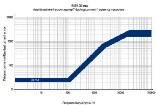
Diagramme FI-/LS-Kombinationen DRCBO 4 Typ B SK, 3+N-polig
