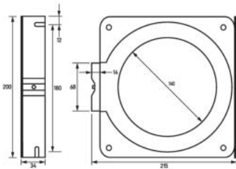
Maßzeichnung Gruppenansicht
