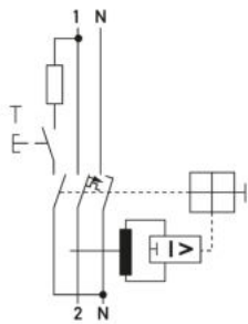
Schaltungsbeispiel FI-/LS-Kombinationen DRCBO 3 Typ AC, B-Charakteristik, 1+N-polig
