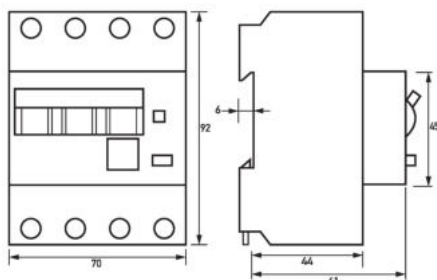
Maßzeichnung FI-/LS-Kombinationen DRCBO 4 Typ A, 3+N-polig
