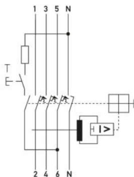
Schaltungsbeispiel FI-/LS-Kombinationen DRCBO 4 Typ A, 3+N-polig
