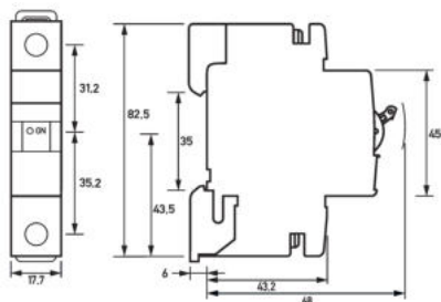
Maßzeichnung Leitungsschutzschalter DLS 6i, Z-Charakteristik, 10 kA
