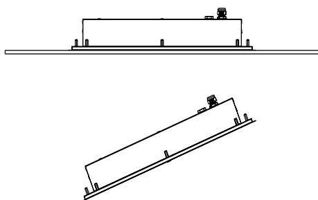
Usazení svítidla BORDER do podhledu
