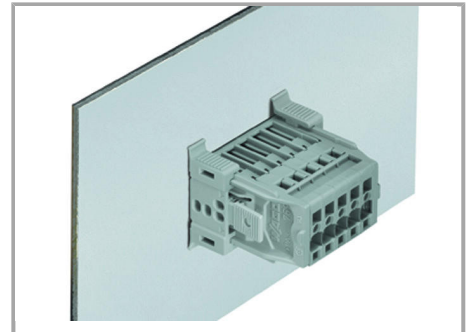
Stilleiste mit Snap-In-Flanschen (769-605 /006-000) im Blechausschnitt
