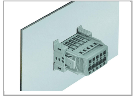
Stilleiste mit Snap-In-Flanschen (769-605/006-000) im Blechausschnitt
