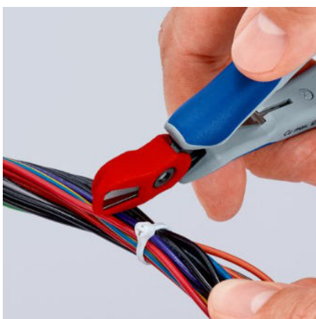
Snadné připevnění: zachytávač materiálu lze snadno a bezpečně připevnit k hlavě kleští
