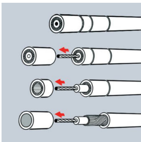
Třístupňové odizolování koaxiálního kabelu
