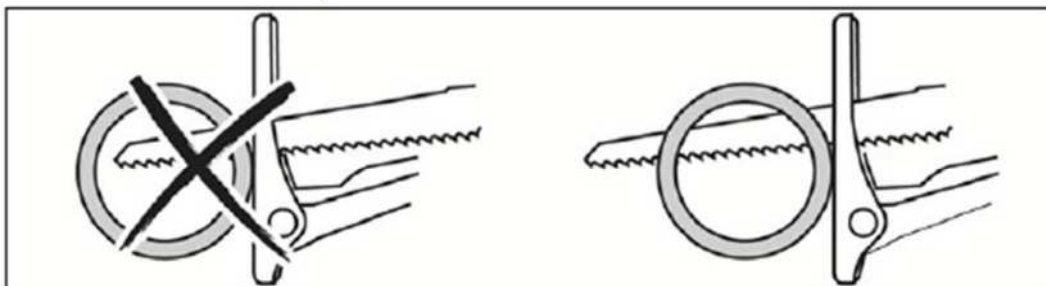
● Oporná patka musí byť zaprená o ťazaný materiál
