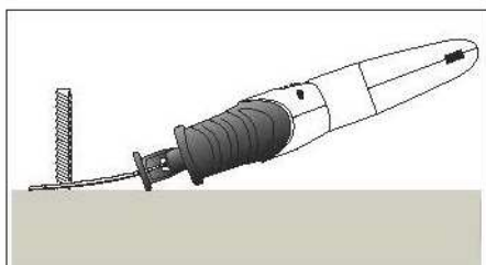
Odčezávaní priamo u stěny
