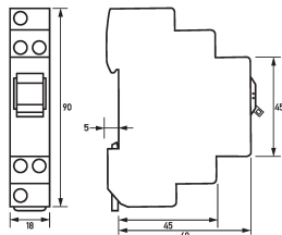
Maßzeichnung Gruppenansicht
