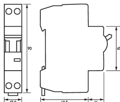
Maßzeichnung Gruppenansicht
