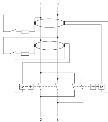
Anschlussschema
