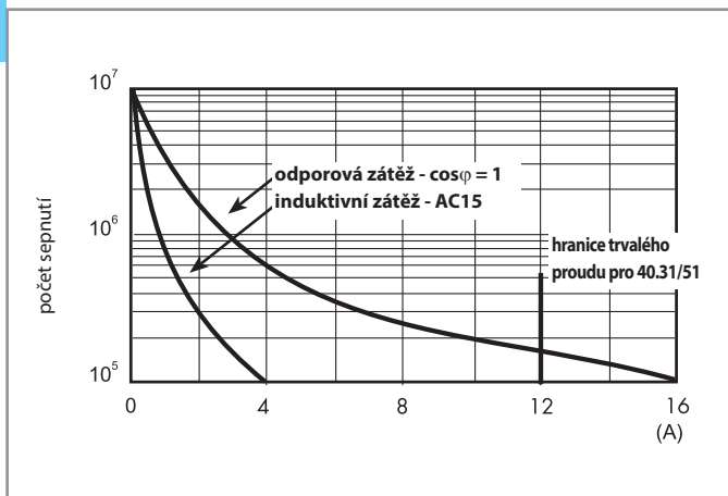
F 40.3 - elektrická životnost při AC typ 40.31/51/61 (strana 4)
