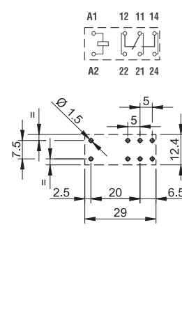
pohled ze strany vývodů
