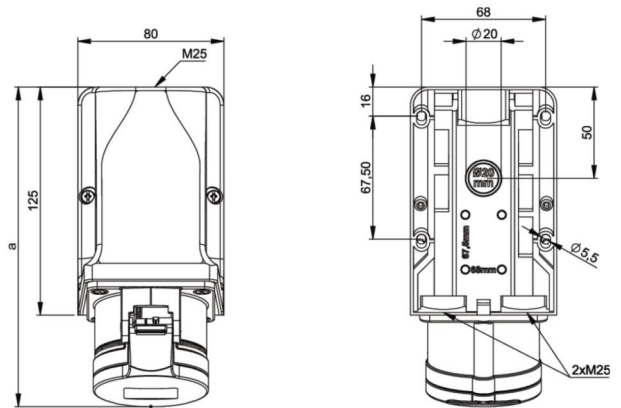
b=Höhe/height Neigung/angle=15°
